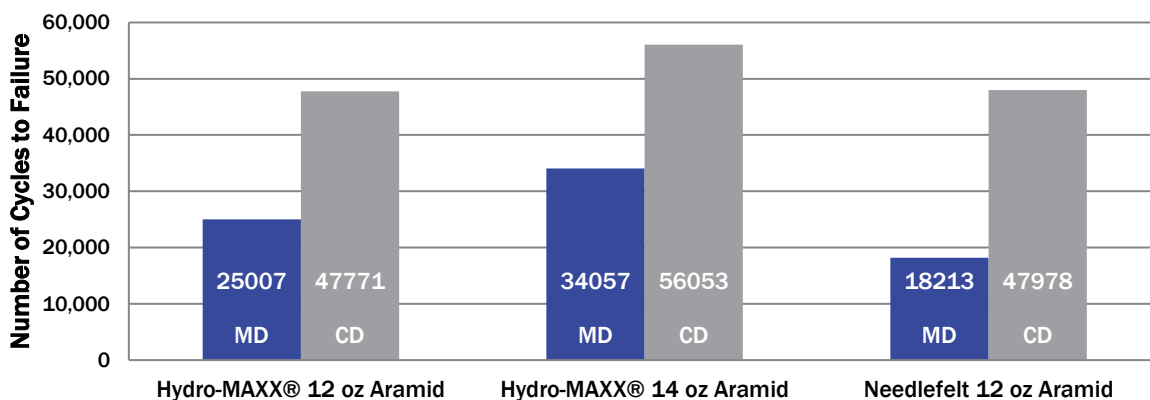
MIT Flex Test Results from ETSI ASTM 02176
